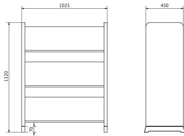
ART.NR E31009 – SNOWFLAKE 950, MED BEN, VIT LAMINAT ITEM NO. E31009 – SNOWFLAKE 950, WITH LEGS, WHITE LAMINATE N° RÉF E31009 – SNOWFLAKE 950, SUR PIEDS, STRATIFIÉ BLANC ART.-NR. E31009 – SNOWFLAKE 950, MIT FÜSSEN, WEISSES LAMINAT
